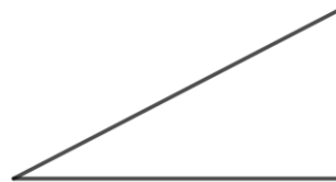
直角三角形
